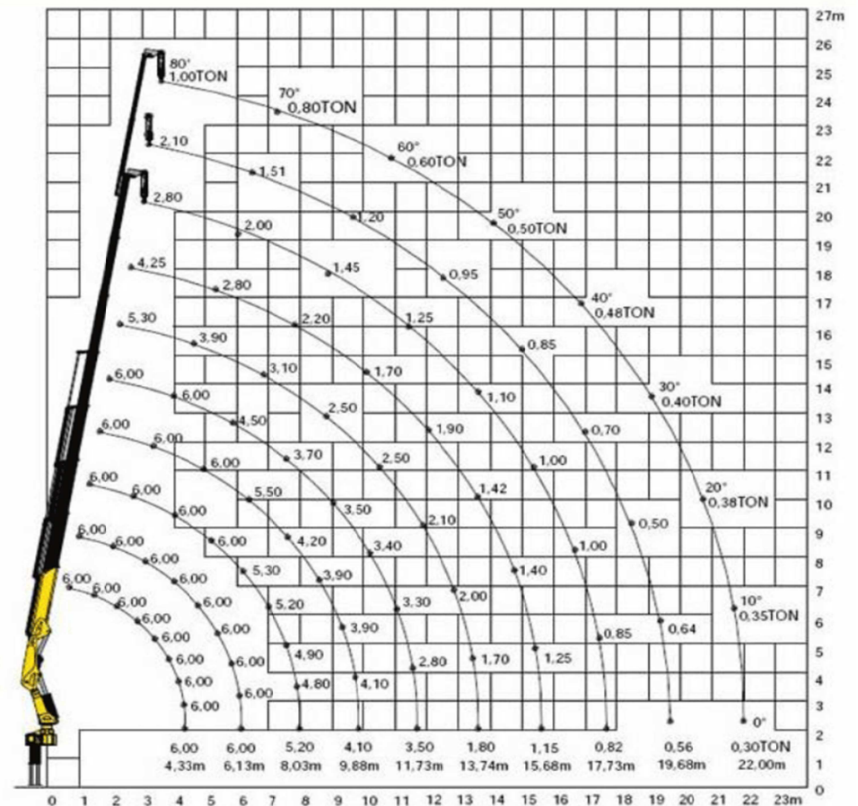
GRÁFICO DE CARGA COM JIB
