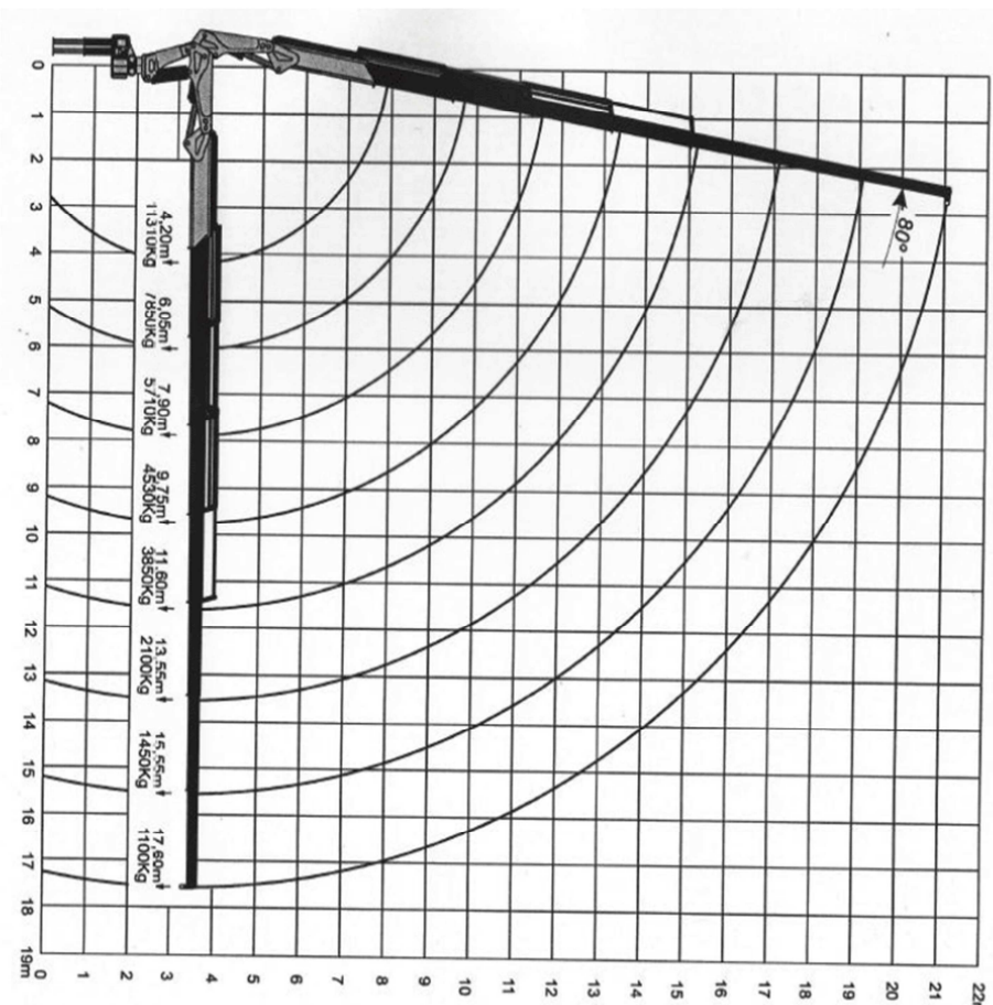
GRÁFICO DE CARGA
