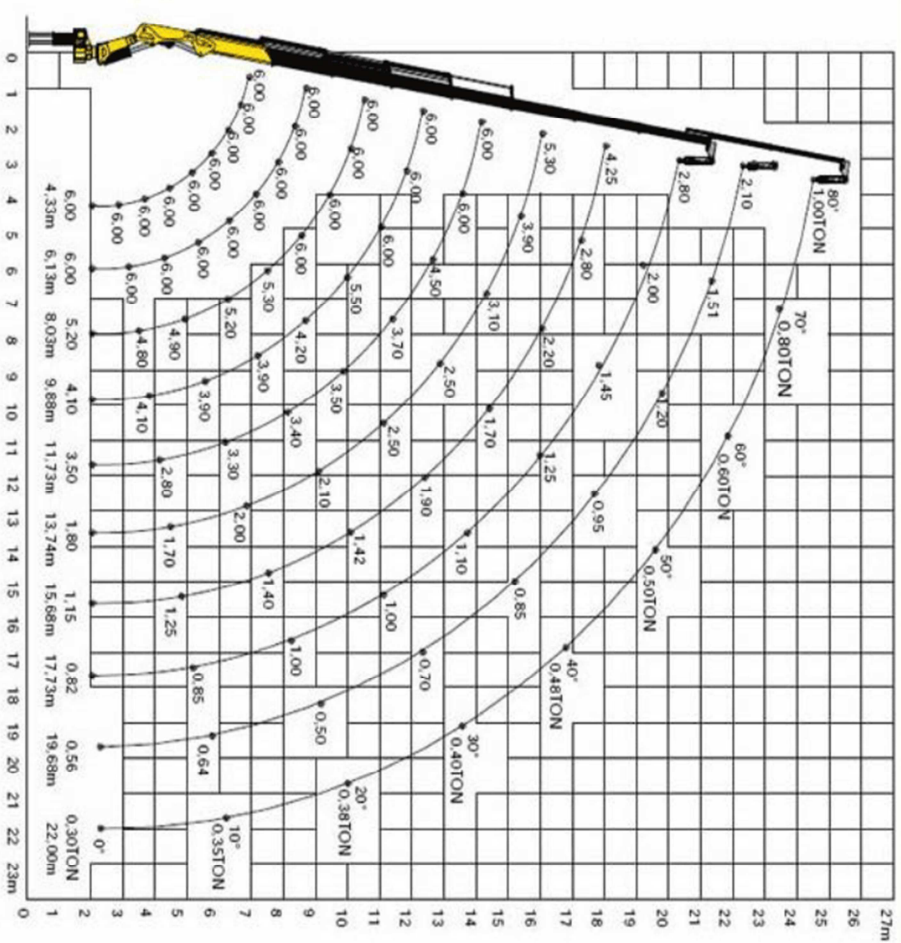
GRÁFICO DE CARGA COM JIB
